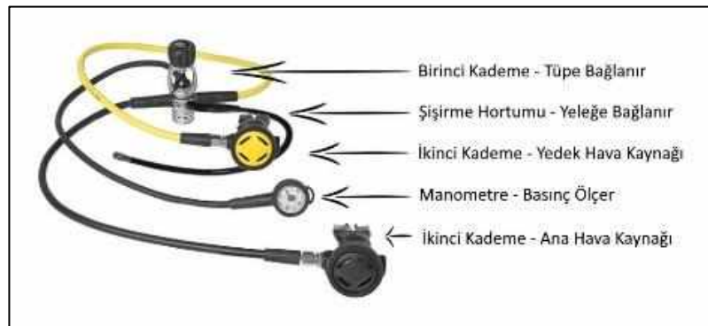
Şekil 4 - Regülatör
